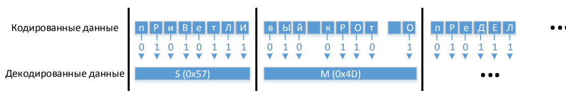
Рис.1. Сдвиговые операции
