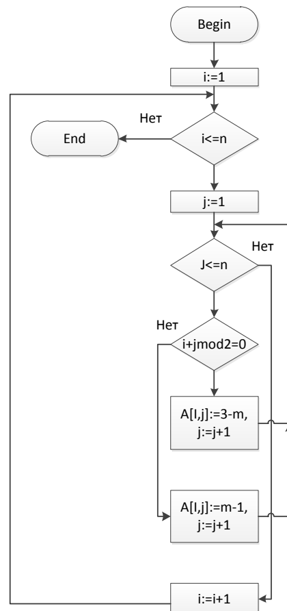
Рис. 2. Блок-схема алгоритма
